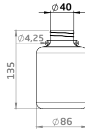
LGM625 Plastic 0,5 L
