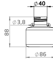
LGM625 Plastic 0,25 L
